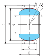
GEG...XT-2RS
