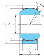
GEG...ET-2RS
