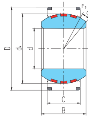
外形尺寸mm
